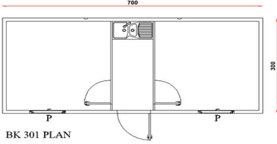
BK 301 PLAN
